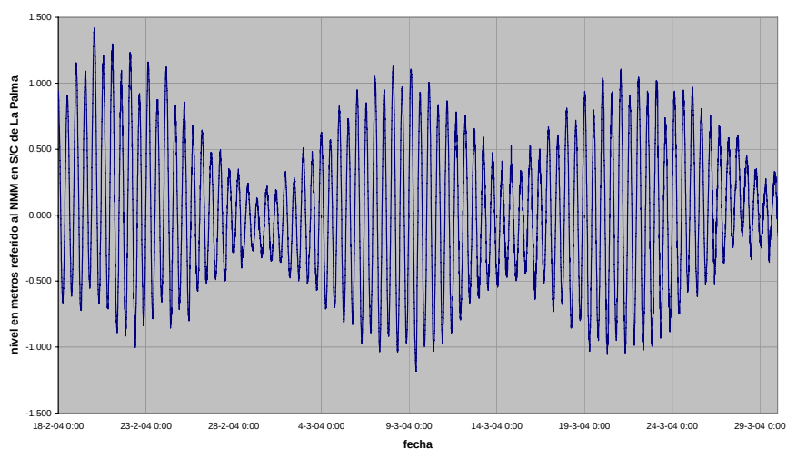
REGISTRO DEL MAREÓGRAFO DE BARLOVENTO
