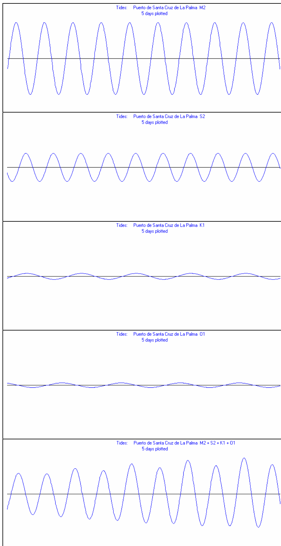
Figura 8.- Representación gráfica de los armónicos M2, S2, K1 y O1 y su sumatorio para La Palma (generado con TPHA, Dalrymple R., Center for Applied Coastal Research, University of Delaware)
