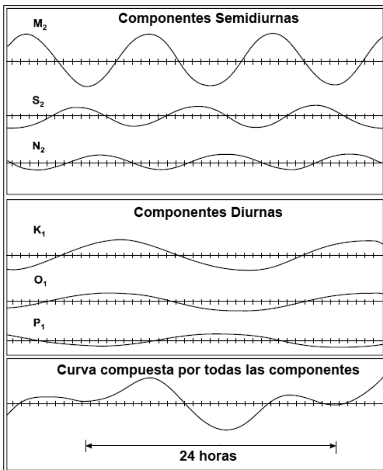
Figura 3.- Representación gráfica de las componentes armónicas principales de las mareas (a partir de Waves, Tides and Shallow-Water Processes, Open University, Butterworth-Heinemann, 2001)
