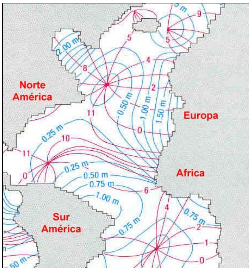
Figura 4.- Puntos anfídromicos en el Atlántico, líneas comareales (ro.) y de amplitud de marea (az.) (a partir de Waves, Tides and Shallow-Water Processes, Open University, Butterworth-Heinemann, 2001)
