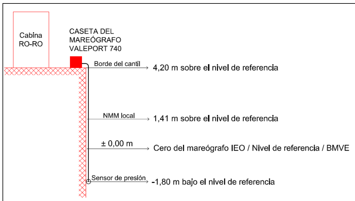
Figura 30.- Esquema de cotas para el Valeport 740 reducido al nivel de referencia del estudio
