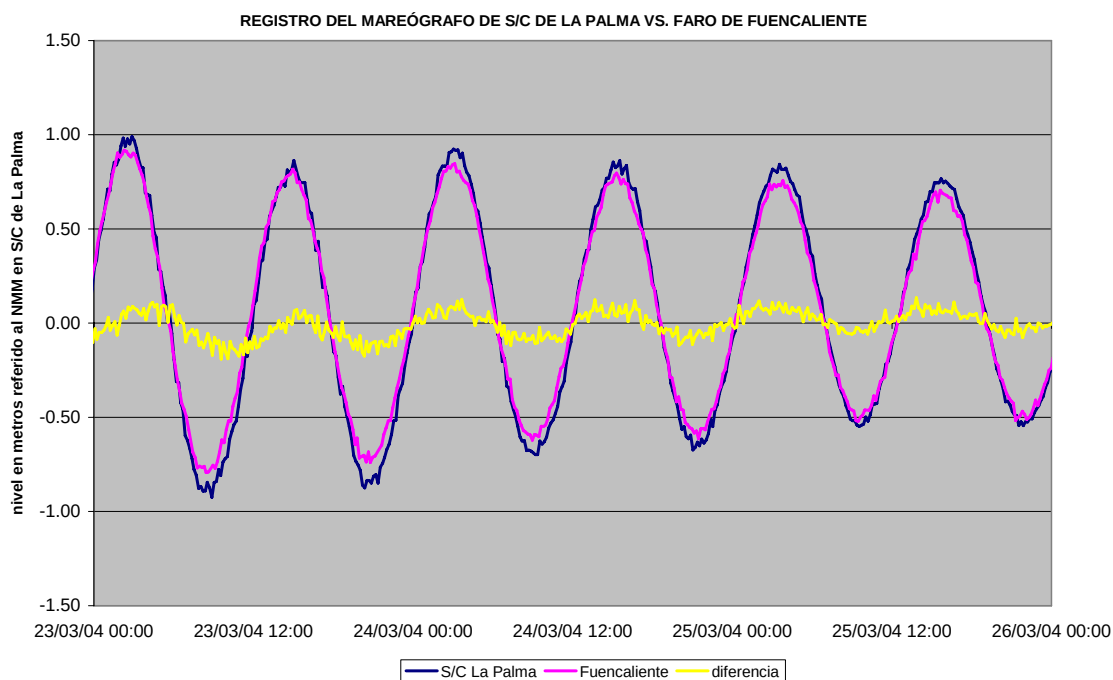
Figura 23.- S/C de La Palma vs. Faro de Fuencaliente en mareas vivas
