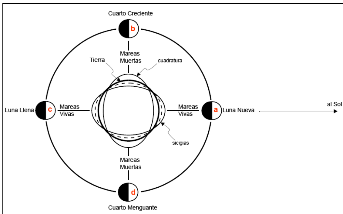
Figura 2.- Diagrama de interacción de las mareas solares y lunares (a partir de Waves, Tides and Shallow-Water Processes, Open University, Butterworth-Heinemann, 2001)
