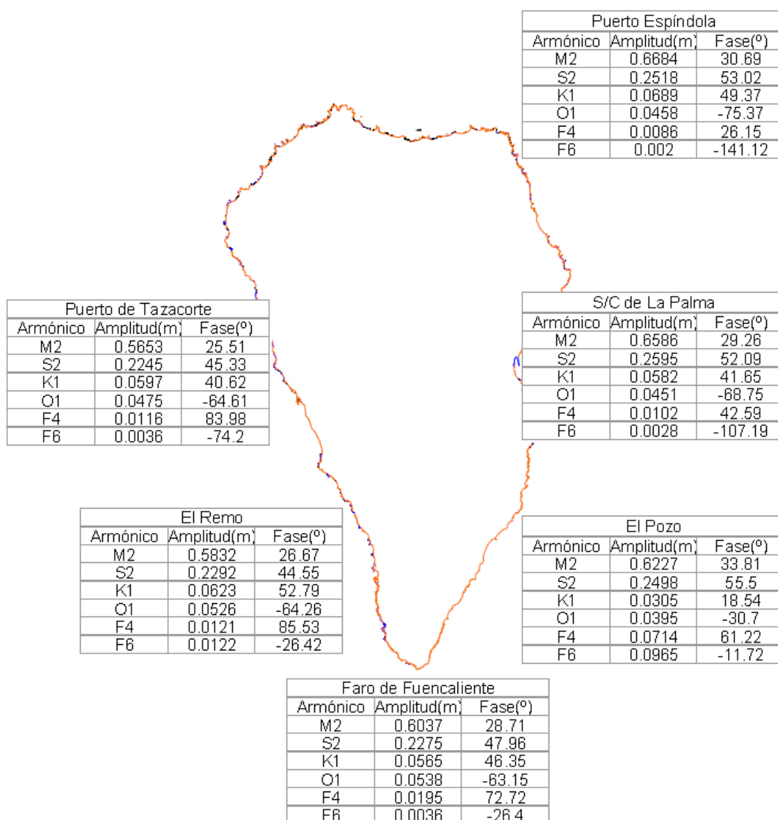
Figura 9.- Armónicos de marea a lo largo del litoral de La Palma
