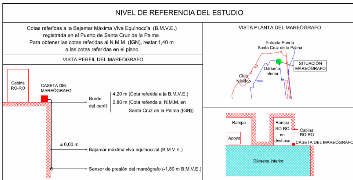
Figura 10.- Localización y referencias del mareógrafo Valeport740
