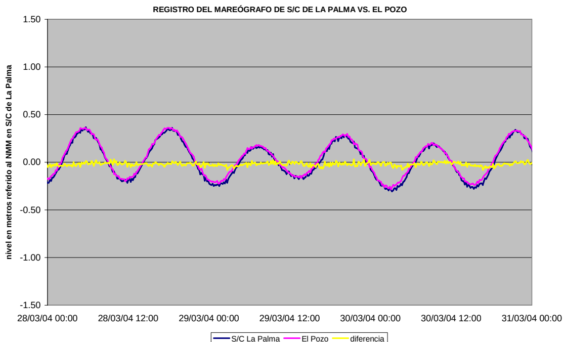
Figura 22.- S/C de La Palma vs. El Pozo en mareas muertas
