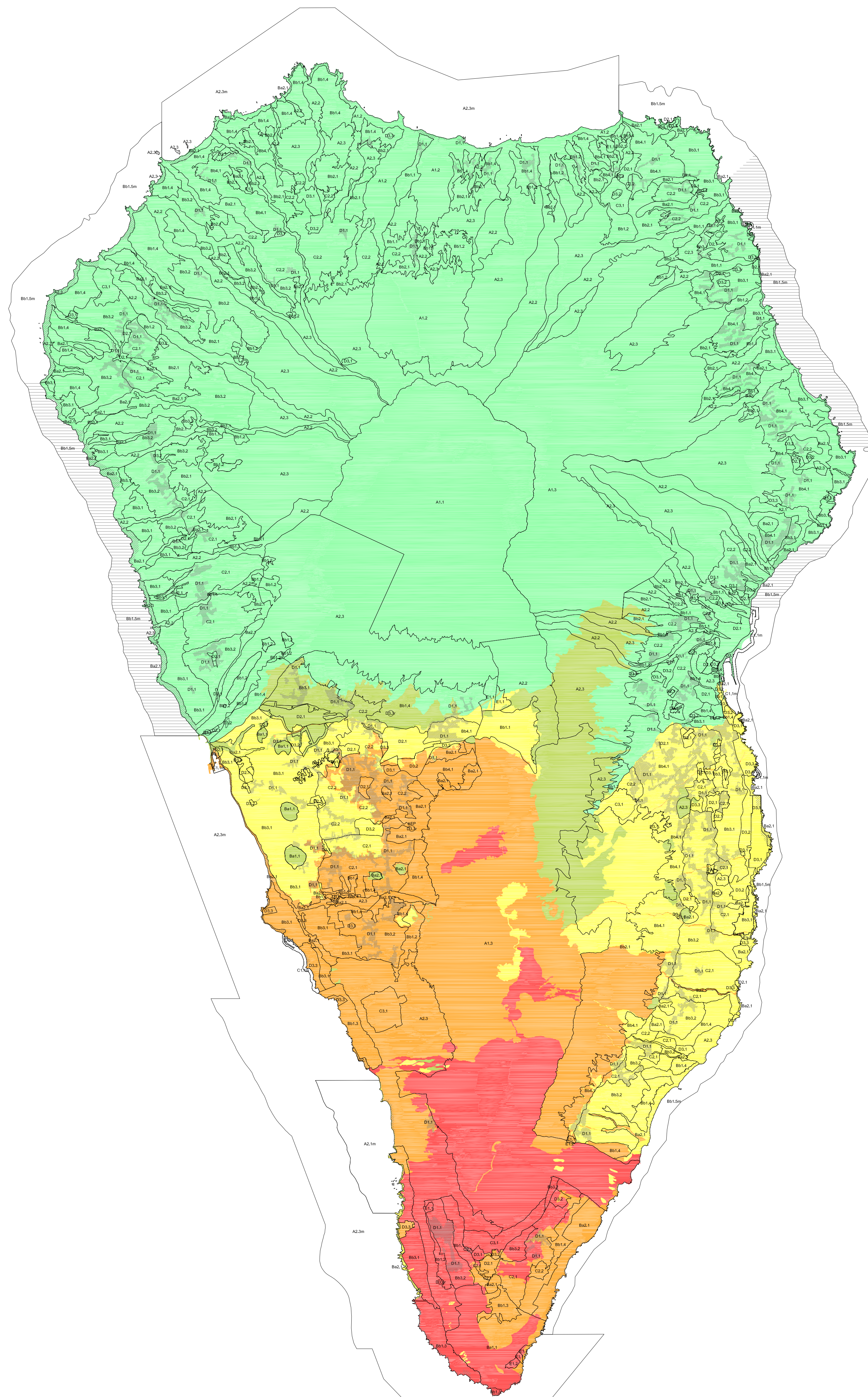
Suceptibilidad Volcánica
