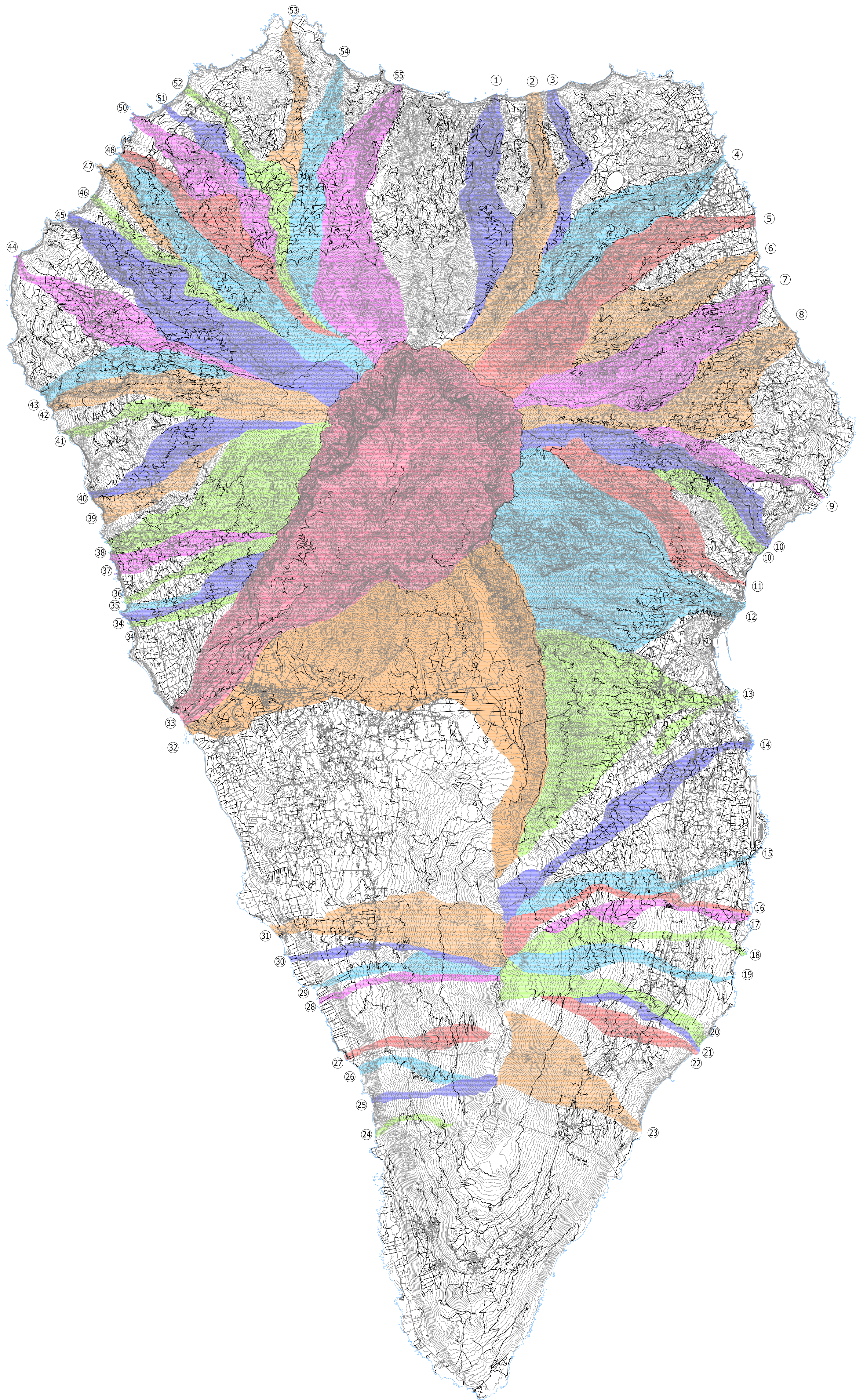
RED HIDROGRÁFICA Y CUENCAS VERTIENTES
