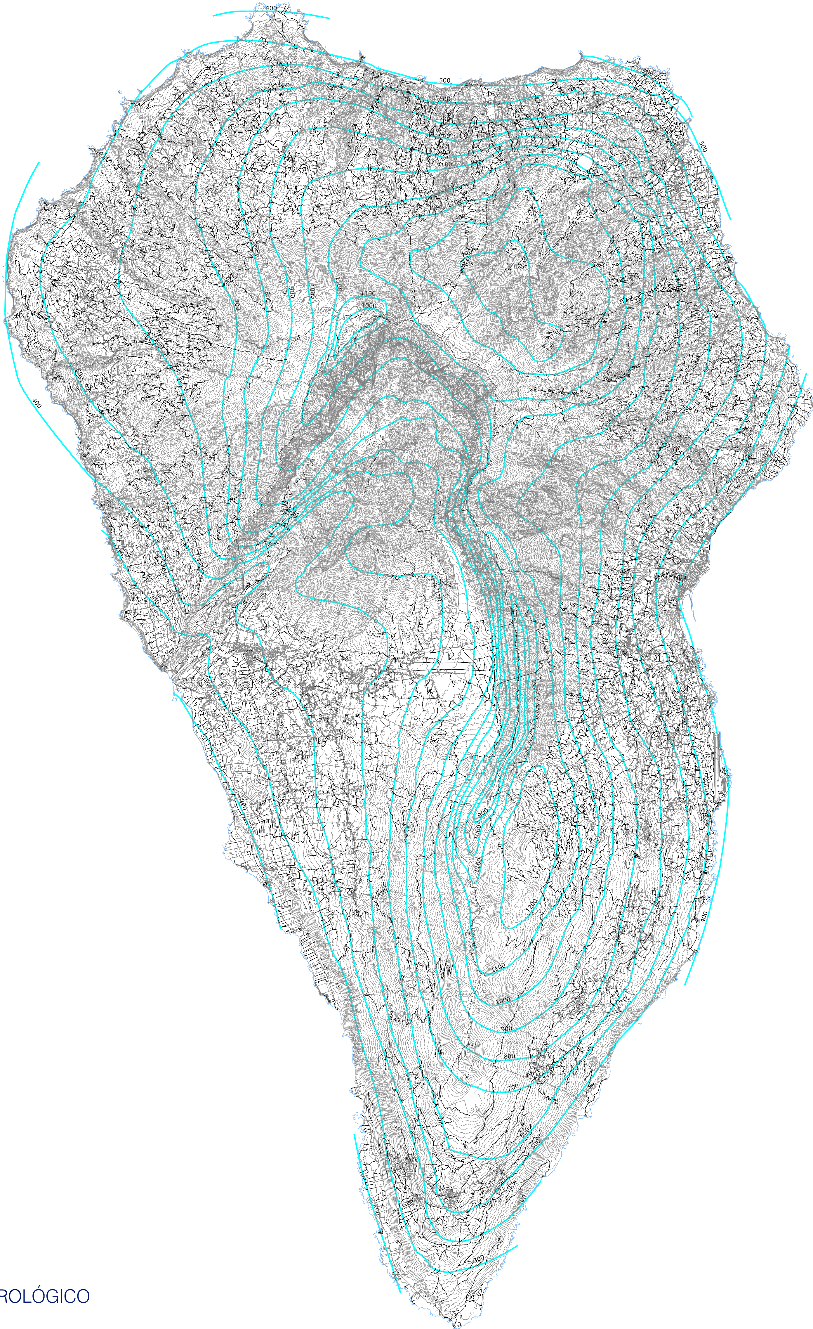
ISOYETAS
